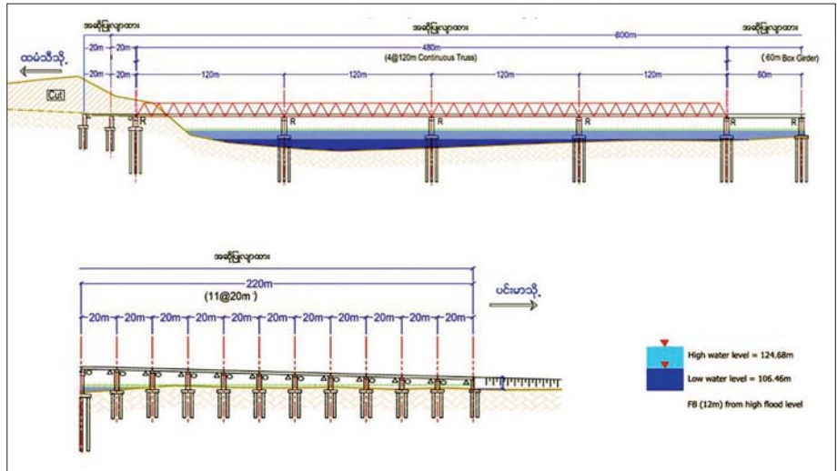
ချင်းတွင်းတံတား (ထမံသီ) အဆိုပြု တံတားပုံစံ။
