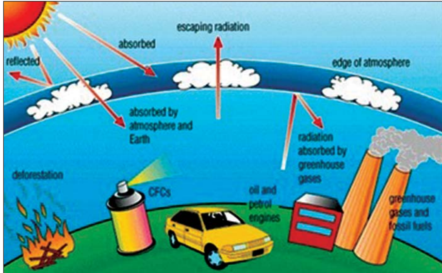
အိုဇုန်းလွှာကို ပျက်စီးစေသော လူသားတို့၏ အသုံးအဆောင်ပစ္စည်းများကို သရုပ်ဖော်ထားပုံ
