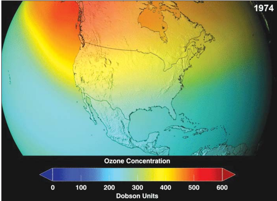
ကလိုရိုဖလူရိုကာဗွန်ကို မဝိတ်ပင်ပါက စထရာတိုစဖီးယားအလွှာမှ အိုဇုန်းစိုးရိမ်မှတ်ကို သရုပ်ဖော်ထားပုံ
