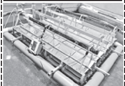
အစွဲအနွယ်ရှိ Solaris Synergy ကုမ္ပဏီ အင်ဂျင်နီယာ များက ရေမျက်နှာပြင်ပေါ်၌ တပ်ဆင်ထားနိုင်သော ဆိုလာပြား များကို သုတေသန ပြုလုပ်ခဲ့စဉ်။ (ဓာတ်ပုံ-အင်တာနက်)
