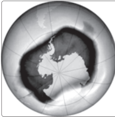
ကမ္ဘာ့အိုစန်းလွှာ ပါးလွှာမှုအနေအထားကို ပြိုဟ်တုမှရိုက်ယူထားသော ဓာတ်ပုံအရ ဤသို့ တွေ့ရသည်။
