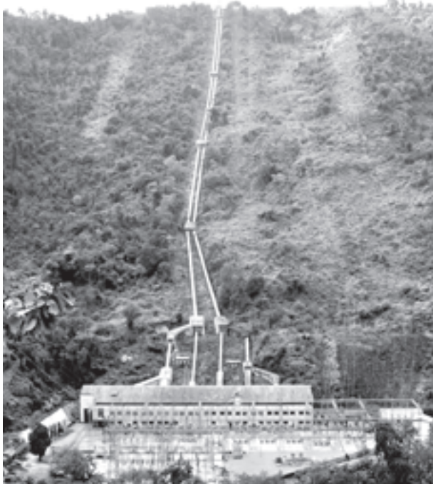
ဘီလူးချောင်း အမှတ်(၂) ရေအားလျှပ်စစ်ဓာတ်အားပေးစက်ရုံ အဆောက်အအုံကြီးနှင့် တောင်ကြောပေါ်၌ သွယ်တန်းထားသောဖိအားမြင့် ပိုက်လိုင်းနှစ်ခုကို တွေ့ရစဉ်။
