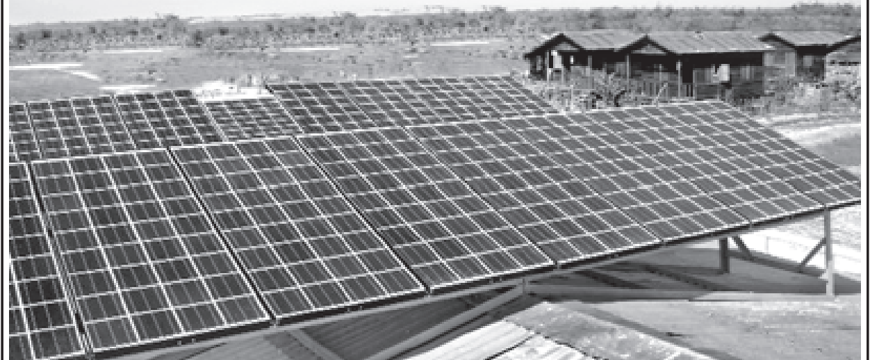
မြင်းခြံမြို့နယ် အရှေ့မြောက်ဘက် ၁၂ မိုင်ခန့်အကွာရှိ ရွာသာယာကျေးရွာတွင် တပ်ဆင်ထားသည့် နေစွမ်းအင်သုံး ဆိုလာပြားများကို ဤသို့ တွေ့ရသည်။
