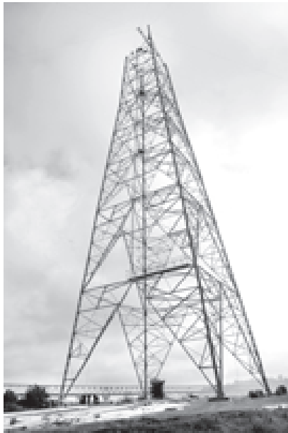
နိုင်ငံတော်ဝန်ကြီးချုပ် ဗိုလ်ချုပ်ကြီးသိန်းစိန် ပန်းတောင်းမြို့နယ် ဧရာဝတီမြစ် အနောက်ဘက်ကမ်း သစ်ဆိမ့်ပင်ကျေးရွာ၌ (၂၃၀)ကေဂျီ ရွှေတောင်-ဥယျာဉ်ပင် မဟာမာတ်အားလှိုင်း ဧရာဝတီမြစ်ကျော် တာဝါတိုင်တည်ဆောက်နေမှုကို ကြည့်ရှု စစ်ဆေးစဉ်။ (သတင်းစဉ်)
