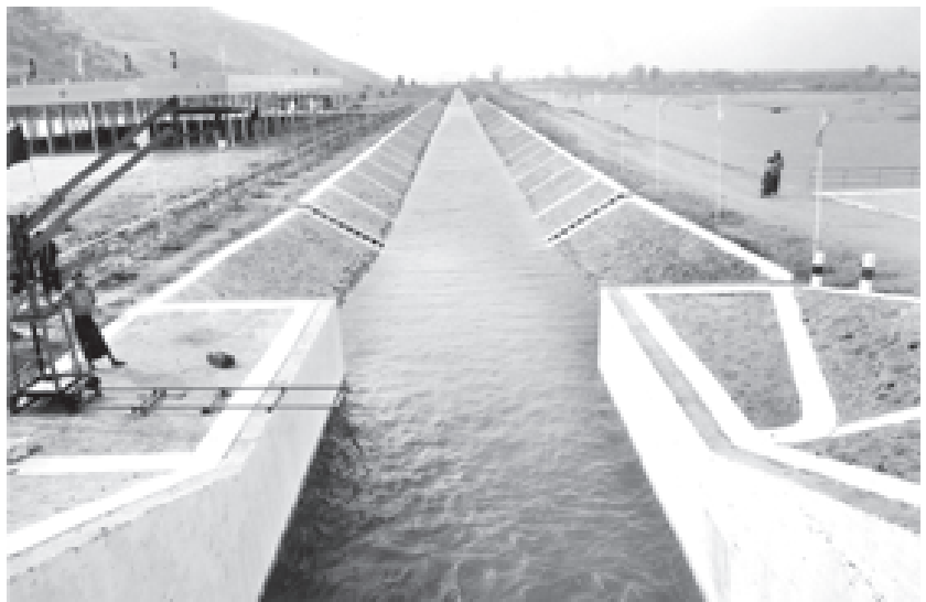
လယ်မြေဧက ၁၆၀၀၀ ကို ဆည်ရေသောက်ပို့လွှတ်မည့် လက်တံမြောင်း ၄၄၄၄ ရှိသော အရှည် ၂၉၁၁၁ မီတာရှိသော ပေါင်းလောင်းရေလွှဲဆည်ကို ဤသို့ တွေ့ရသည်။ (မြန်မာ့အလင်း)
