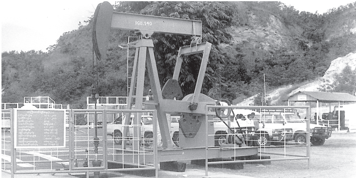
မကွေးတိုင်း ပခုက္ကူခရိုင် ပေါက်မြို့နယ်ရှိ သကြီးတောင် ရေနံမြေနှင့် သဘာဝဓာတ်ငွေ့မြေရှိ ရေနံတွင်းအမှတ်(၁)ကို တွေ့ရစဉ်။ ဓာတ်ပုံမှတ်တမ်း(မြန်မာ့အလင်း)
