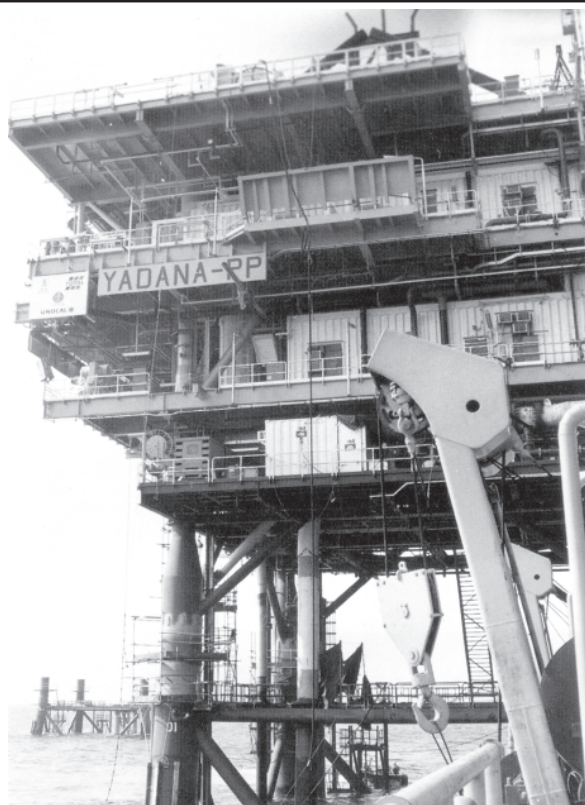
တနင်္သာရီကမ်းရိုးတန်း မုတ္တမကမ်းလွန်တွင် မြန်မာ့ပင်လယ်ပြင်မှ သဘာဝဓာတ်ငွေ့ တူးဖော်ထုတ်လုပ်ခြင်းလုပ်ငန်း ဆောင်ရွက်နေသည့် ရတနာသဘာဝဓာတ်ငွေ့ တူးဖော်ရေးလုပ်ကွက် အမှတ်(၁) ရေနံတူးဖော်စင်ကို ဤသို့ တွေ့ရသည်။ ဓာတ်ပုံမှတ်တမ်း(မြန်မာ့အလင်း)
