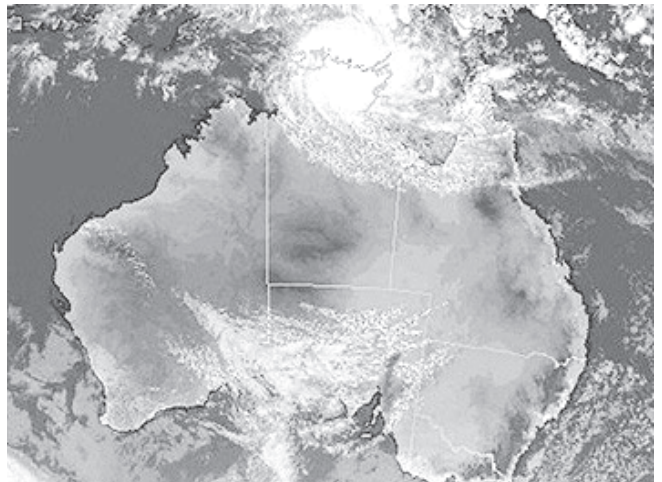
မိုနီကာဆိုက်ကလုန်းမုန်တိုင်း ဝင်ရောက်လာသည့် ဂြိုဟ်တုရုပ်ရိပ် (ဓာတ်ပုံ-အင်တာနက်)
