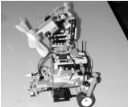
ပြိုင်ပွဲဝင် ဆုရမီးသတ်စက်ရုပ်တစ်ရပ်ကို ဤသို့ တွေ့ရသည်။ (ဓာတ်ပုံ-အင်တာနက်)
