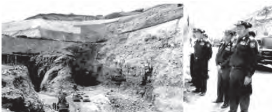
首相梭温与随从视察瑞丽江水电项目的引水隧道建设
