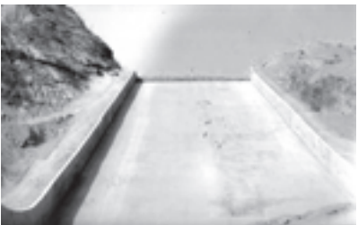
ရေပိုလွှဲကွန်ကရစ်လုပ်ငန်းပြီးစီးမှုကိုတွေ့ရစဉ်။
