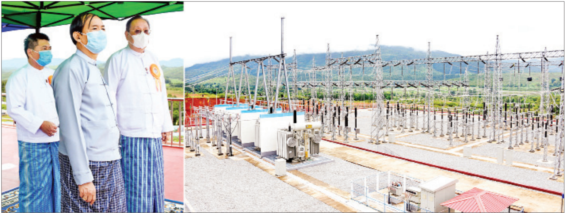
နိုင်ငံတော်သမ္မတ ဦးဝင်းမြင့် ကျိုင်းတုံပင်မဓာတ်အားခွဲရုံ၊ ရှုရပ်နေရာမှ ပင်မဓာတ်အားခွဲရုံ၏ Switch Yard ကို ကြည့်ရှုစဉ်။
