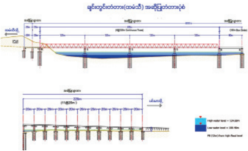
ထပ်မံတည်ဆောက်မည့် ချင်းတွင်းတံတား(ထမံသီ) ပုံစံကို တွေ့ရစဉ်။
