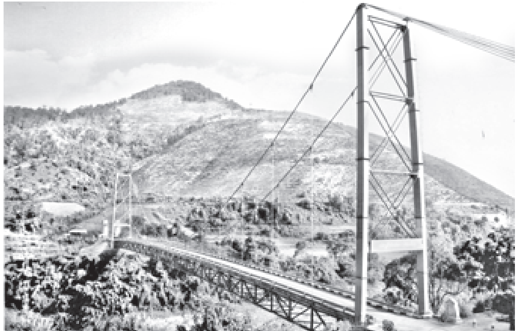
ကွတ်ခိုင်-တာမိုးညး-မိုးစီး-တာပါး-တာရွှေထန်(၇၈)မိုင် လမ်းပေါ်တွင် သံလွင်မြစ်ကူးတံတား တာပါးကို တွေ့ရစဉ်။
