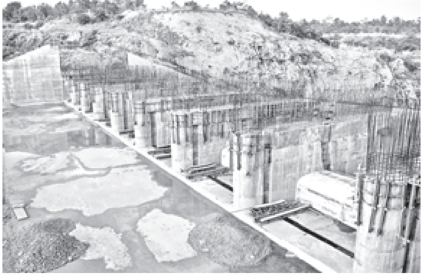
ပြည်တွင်းမြစ် ရေတံခါးများနှင့် ဆက်စပ်ပစ္စည်းများ တပ်ဆင်မည့် ကြီးအုံကြီးဝဲရေလျှောင်တံစီမံကိန်း ရေပိုလွှဲကို တွေ့ရစဉ်။
