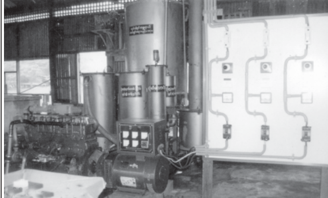
မြန်မာတီထွင်သူများ သမဝါယမအသင်း လီမိတက် က တီထွင်ထုတ်လုပ်သည့် စပါးခွံဓာတ်ငွေ့ထုတ်စက်ဖြင့် လျှပ်စစ်မီးပေးနေလုပ်ငန်း ဆောင်ရွက်နိုင်မှုကို တွေ့ရစဉ်။
