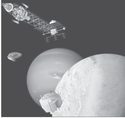
နက်ပီကျွန်းဂြိုဟ် လေ့လာရေး ဂြိုဟ်ဆင်းယာဉ်ပုံစံကို ပန်းချီဆွဲကူး ဖြင့်သရုပ်ဖော်ထားစဉ်။
