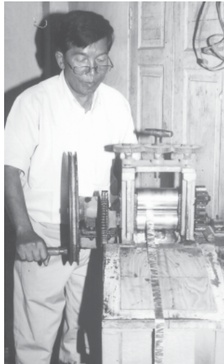
ရွှေဆိုင်းလုပ်ငန်း၏ ပထမအဆင့် အလေးချိန် ၀.၃၁၈၅၇ ကျပ်သားရှိ ရွှေသားကို နန်းကြိတ်စက်ဖြင့် နန်းဆွဲစဉ်။
