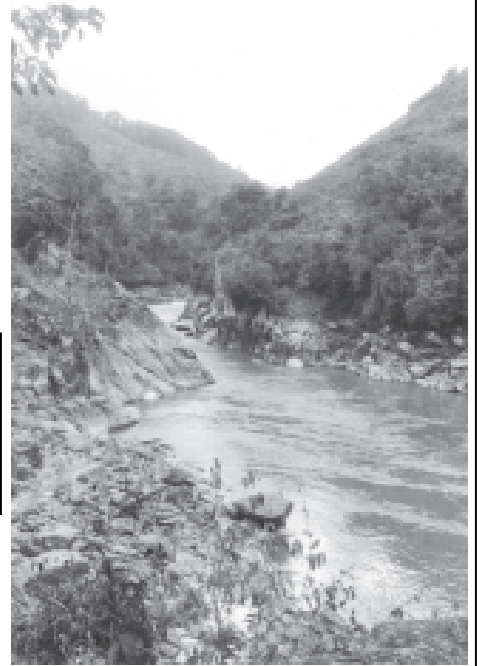
ရှမ်းပြည်နယ် နမ့်ခမ်းမြို့နယ်ရှိ လျှပ်စစ်ဓာတ်အားမဂ္ဂါဝပ် ၄၀၀ ထုတ်ယူရရှိမည့် ရွှေလီရေအားလျှပ်စစ်စီမံကိန်းလုပ်ငန်းမှ ကွန်ကရစ်တံပိတ်မည့် ရွှေလီမြစ်ကျဉ်းနေရာကို တွေ့ရစဉ်။
